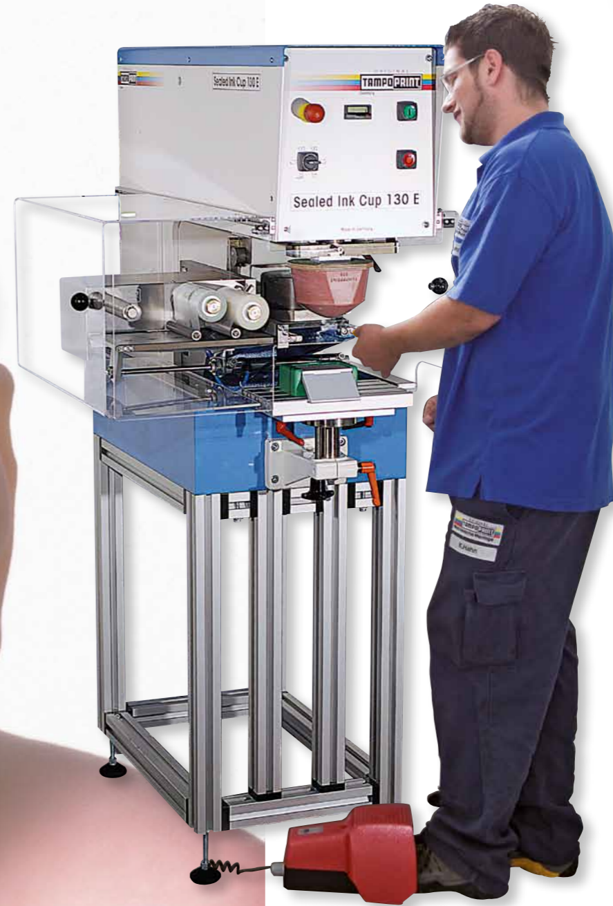
"Sealed Ink Cup 130 E" ve tamamlayıcıları artık silikon temizleme ünitesi, alüminyum profil ayak ve x/y tabla ile tek başına bir çalışma birimi oluşturmaktadır.
